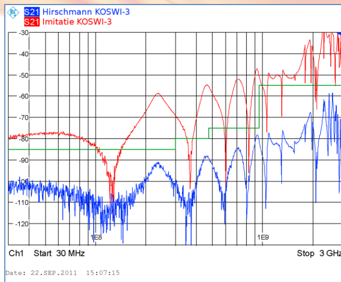
Resultaten EMV-test conform eisen Kabel Keur
